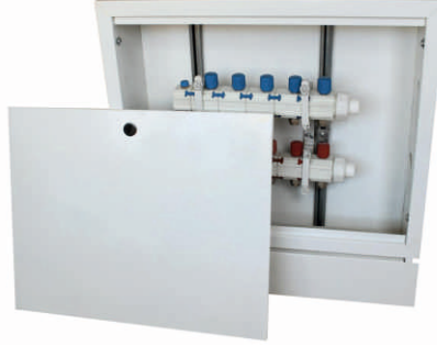
Kollektör Dolabı
